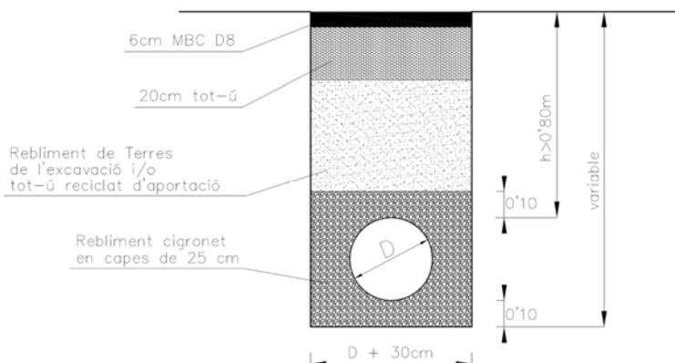
Secció tipus clavegueram
